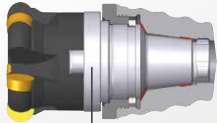
Mit QuickFlex®- Fräsdornaufnahme
