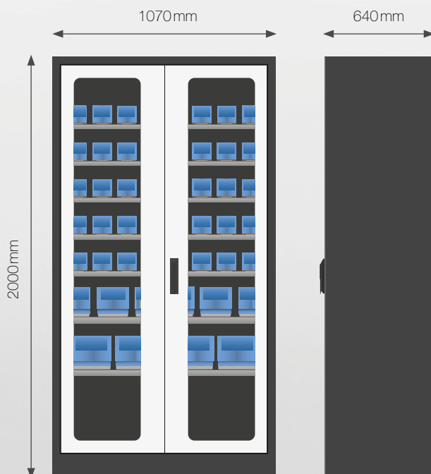
TM 626 mit Sichtfenster | Front- & Seitenansicht
