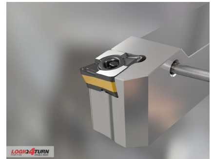
Einfacher Schneidenwechsel durch neuen, seitlichen Klemmmechanismus
