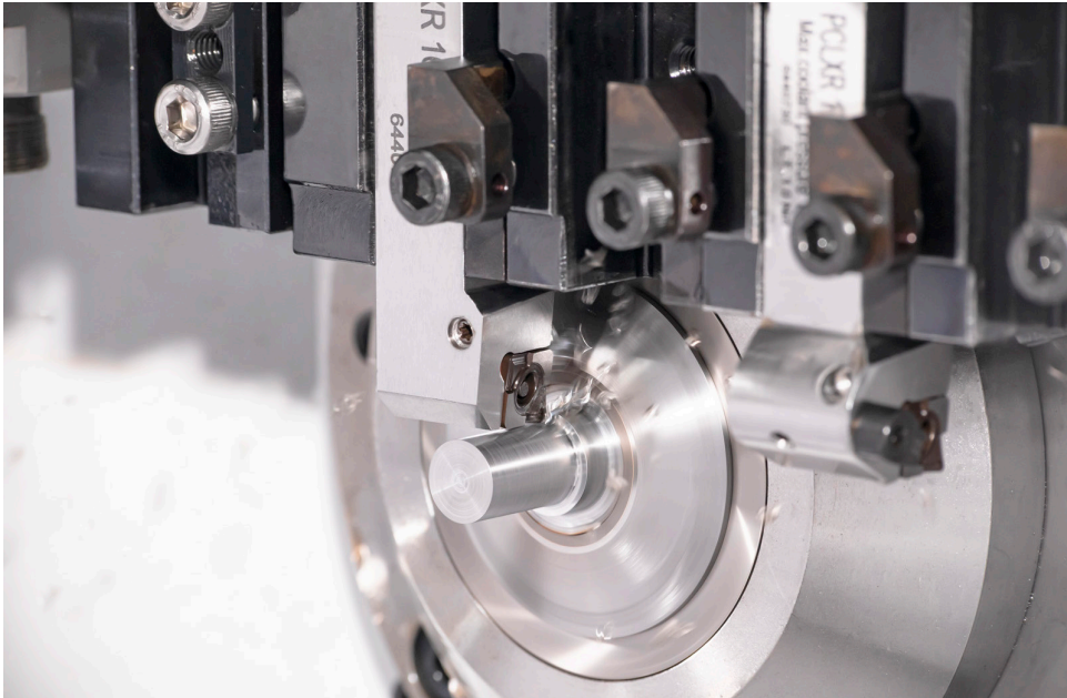
Einfacher Schneidenwechsel durch neuen, seitlichen Klemmmechanismus
